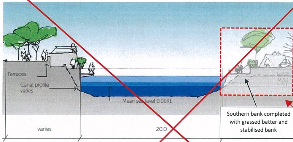
Section A-A – Stage 1a Corso
