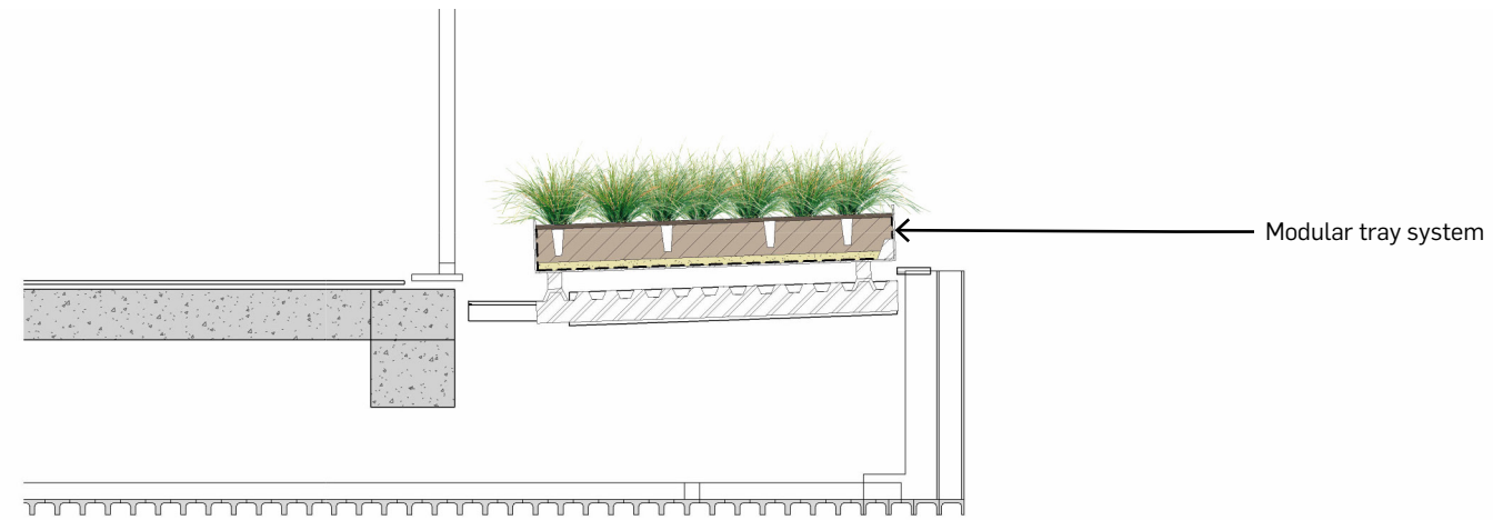
5 Level 1 - Section 5 LS-200-L01-00 1 : 25
