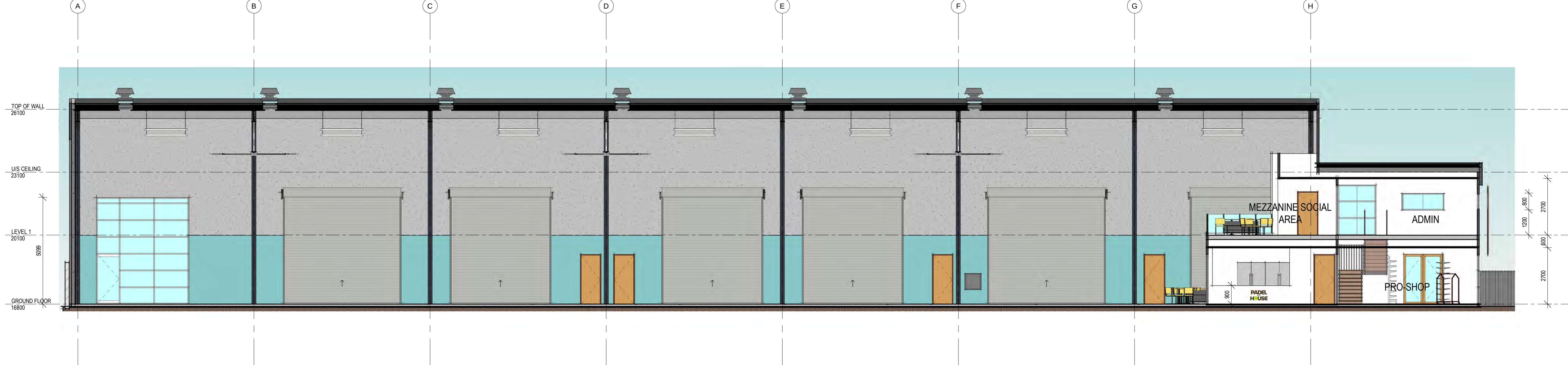
1 SECTION A-A 1 : 100
