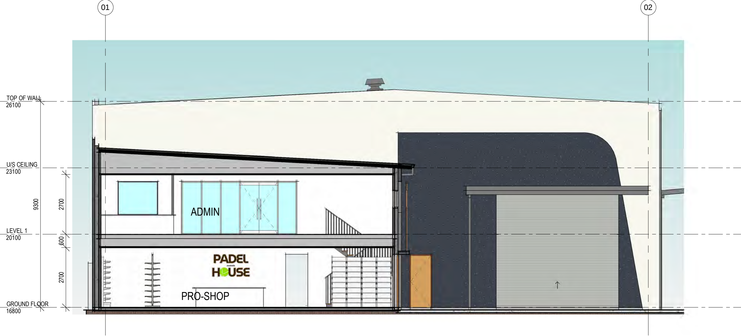
2 SECTION B-B 1 : 100
