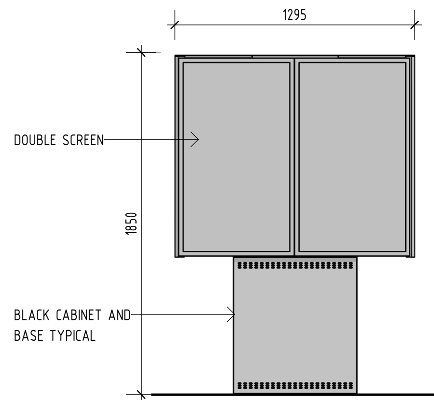
4 S20-A - DOUBLE DIGITAL MENU 1 : 20
