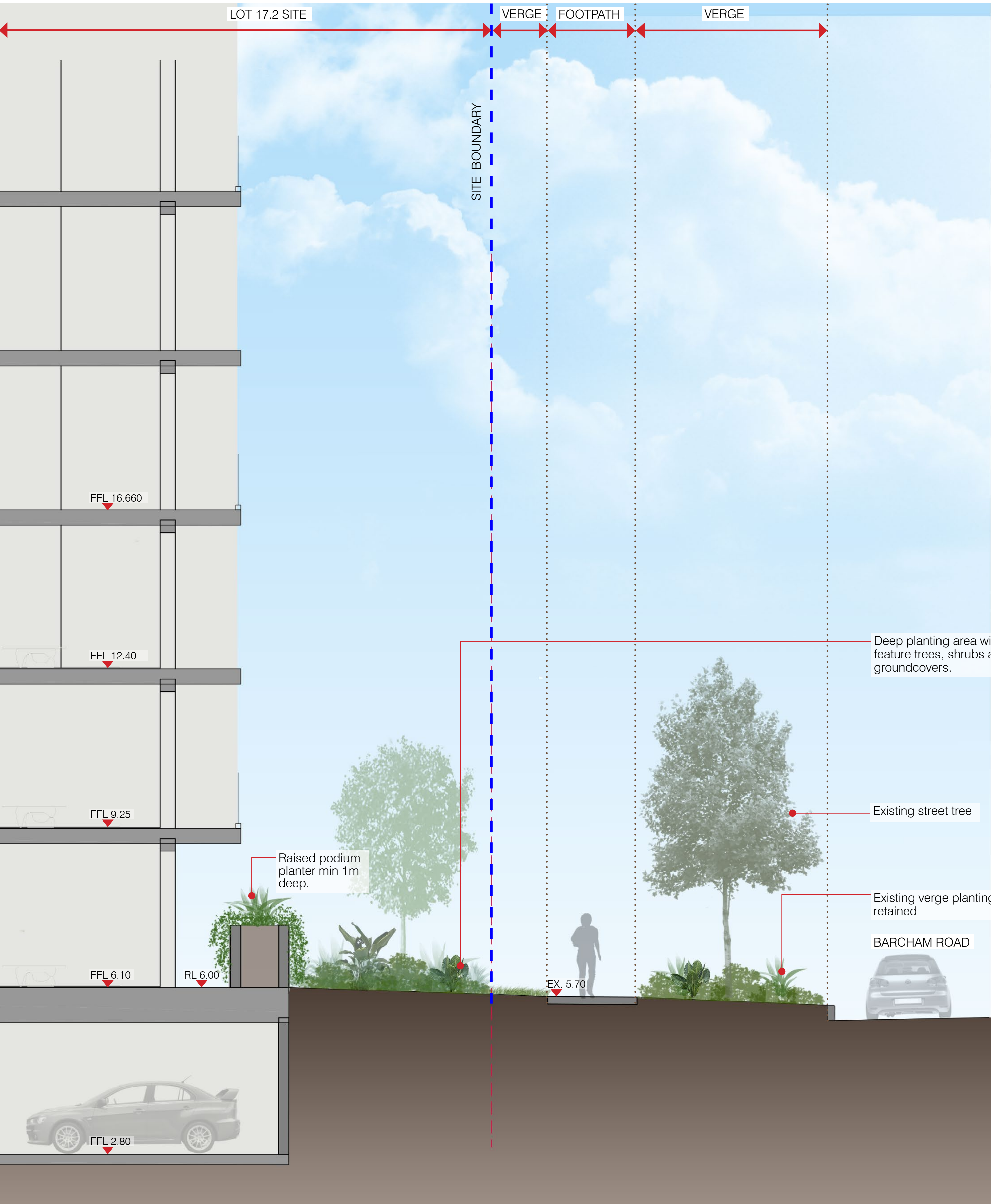
SECTION C 1:50 @ A1
