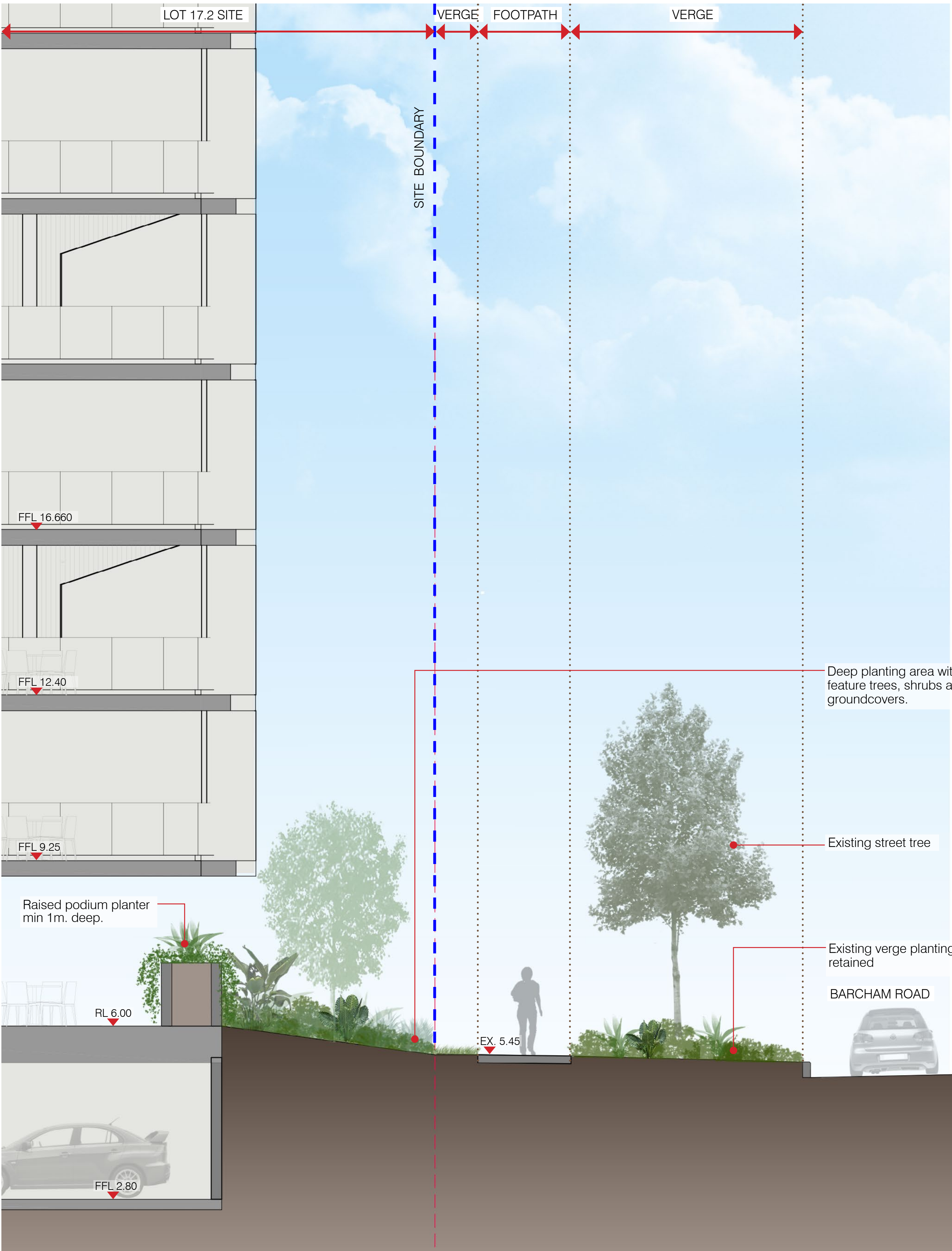
SECTION E 1:50 @ A1
