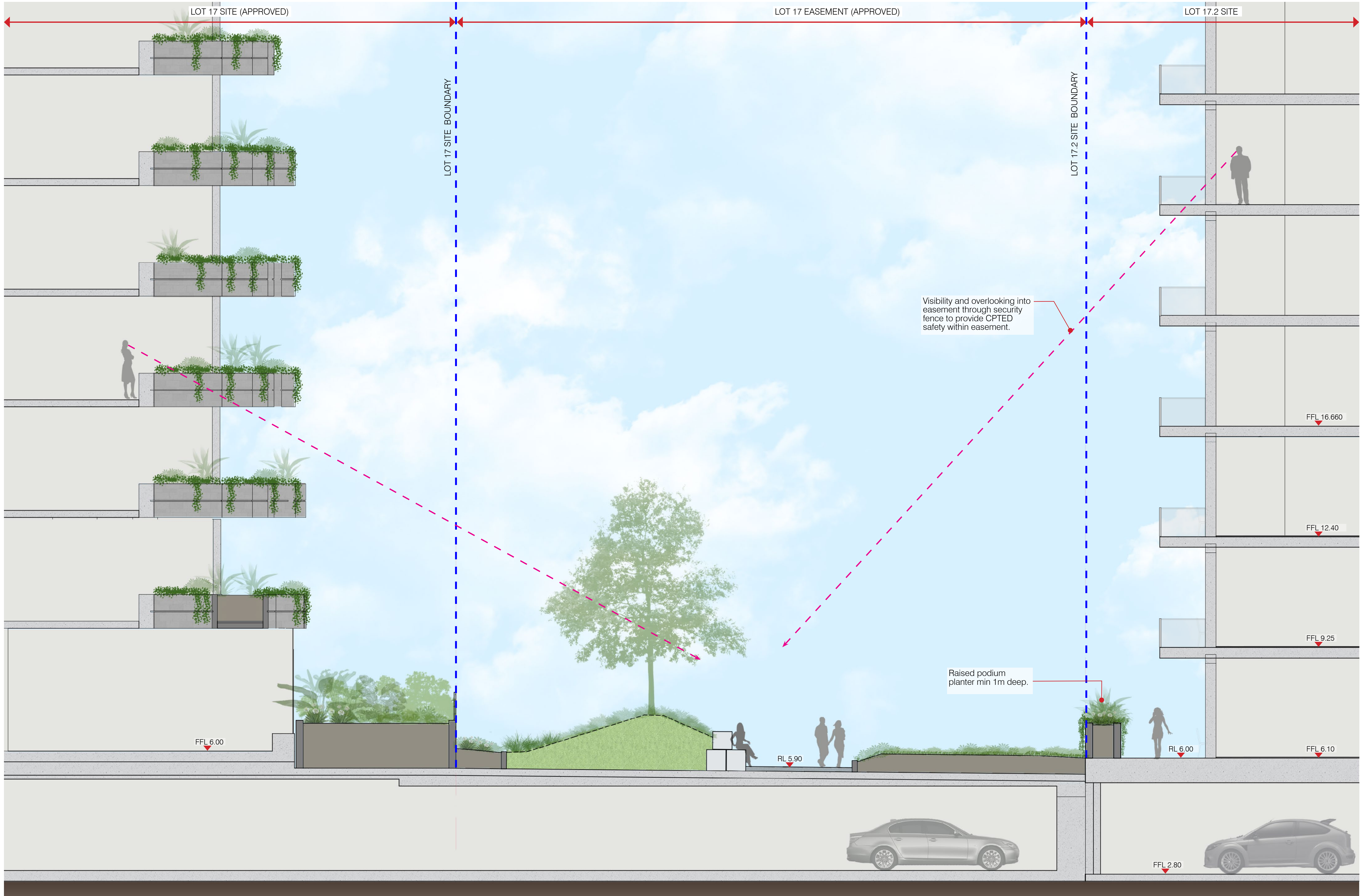
SECTION J 1:50 @ A1
