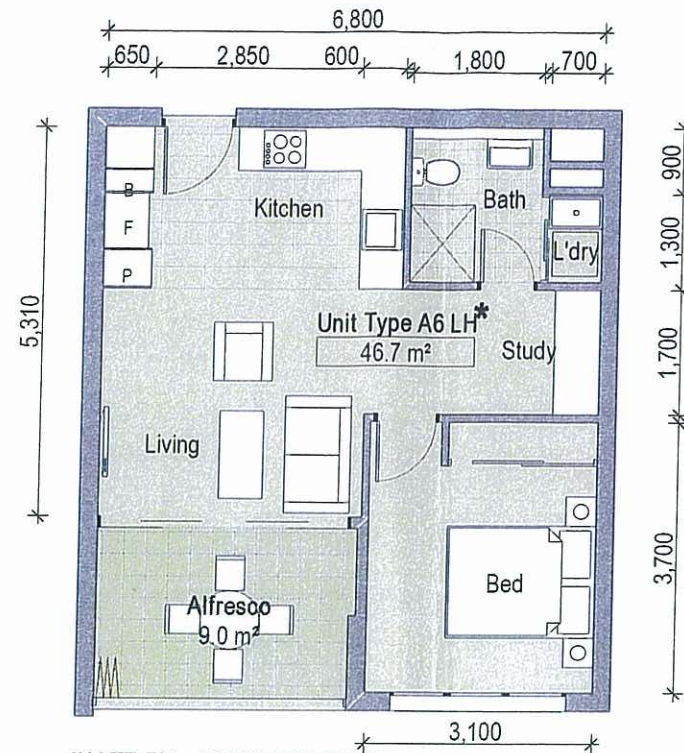
1 Unit A6 SCALE 1:50 @ A1
