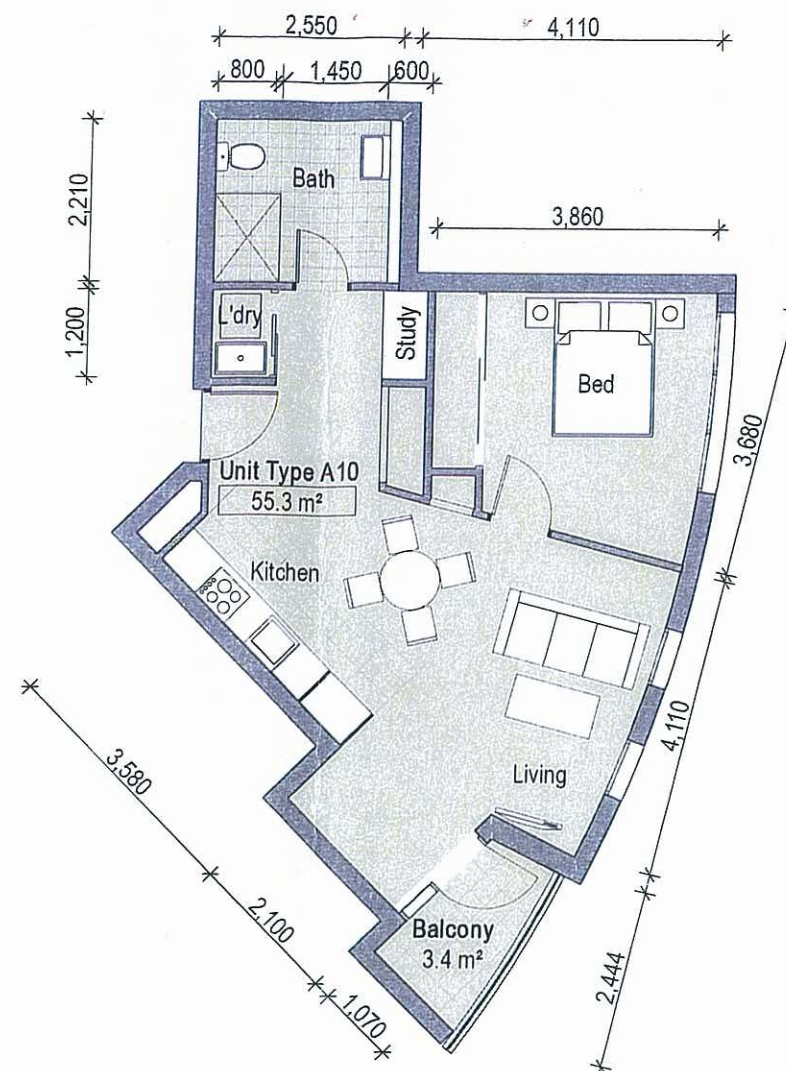
2 Unit A10 SCALE 1:50 @ A1
