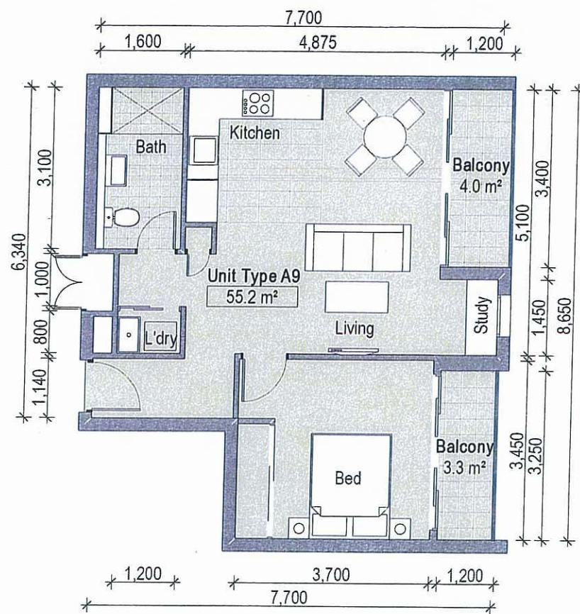
1 Unit A9 SCALE 1:50 @ A1
