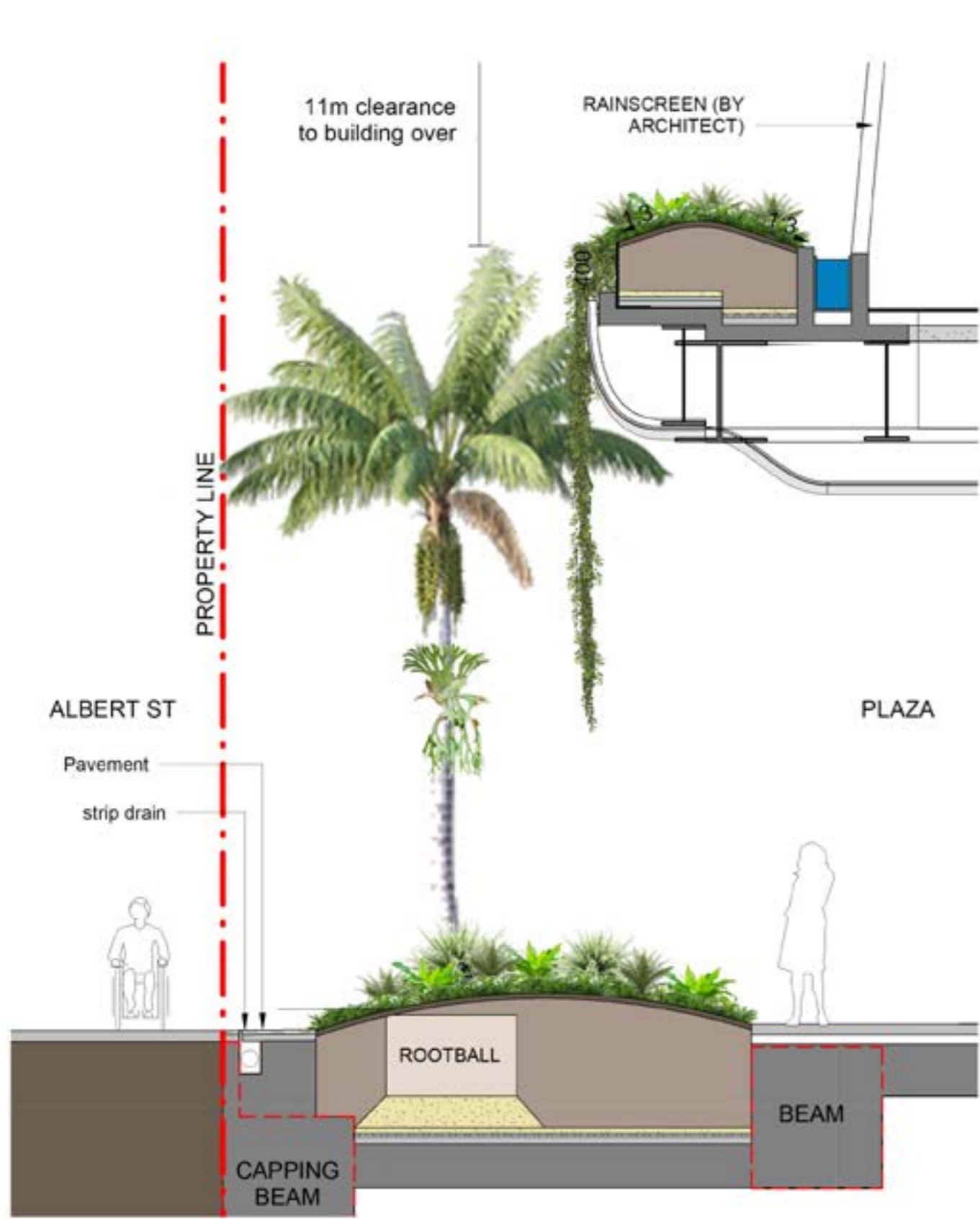
1 Central Planter Section 1 - 1 : 50
