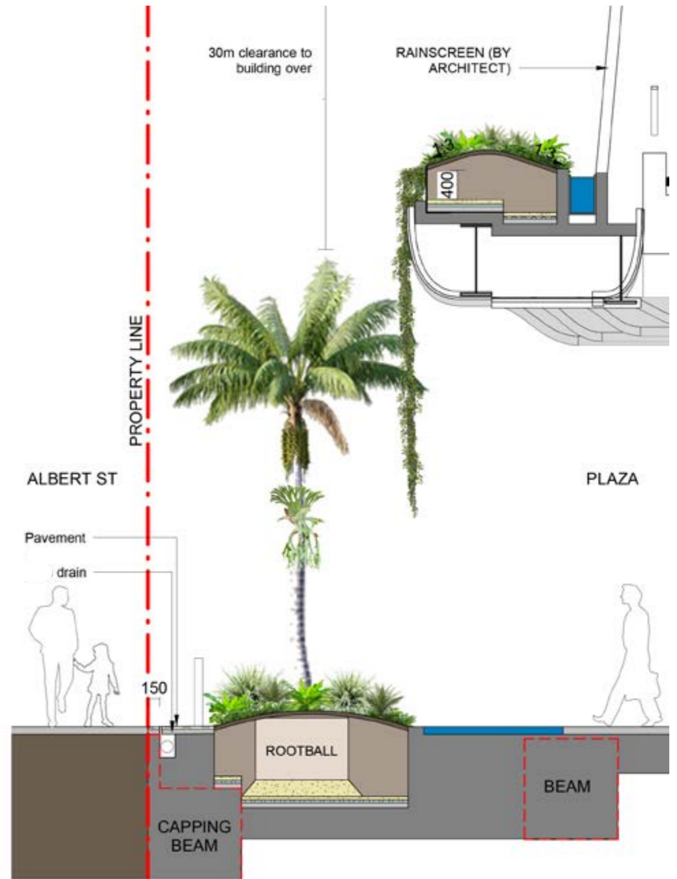
2 Central Planter Section 2 - 1 : 50
