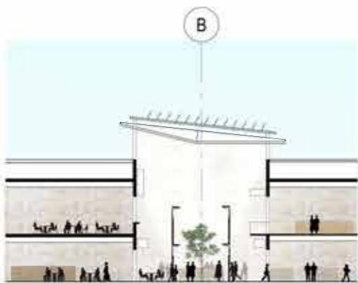
2 SECTION 2 1:250
