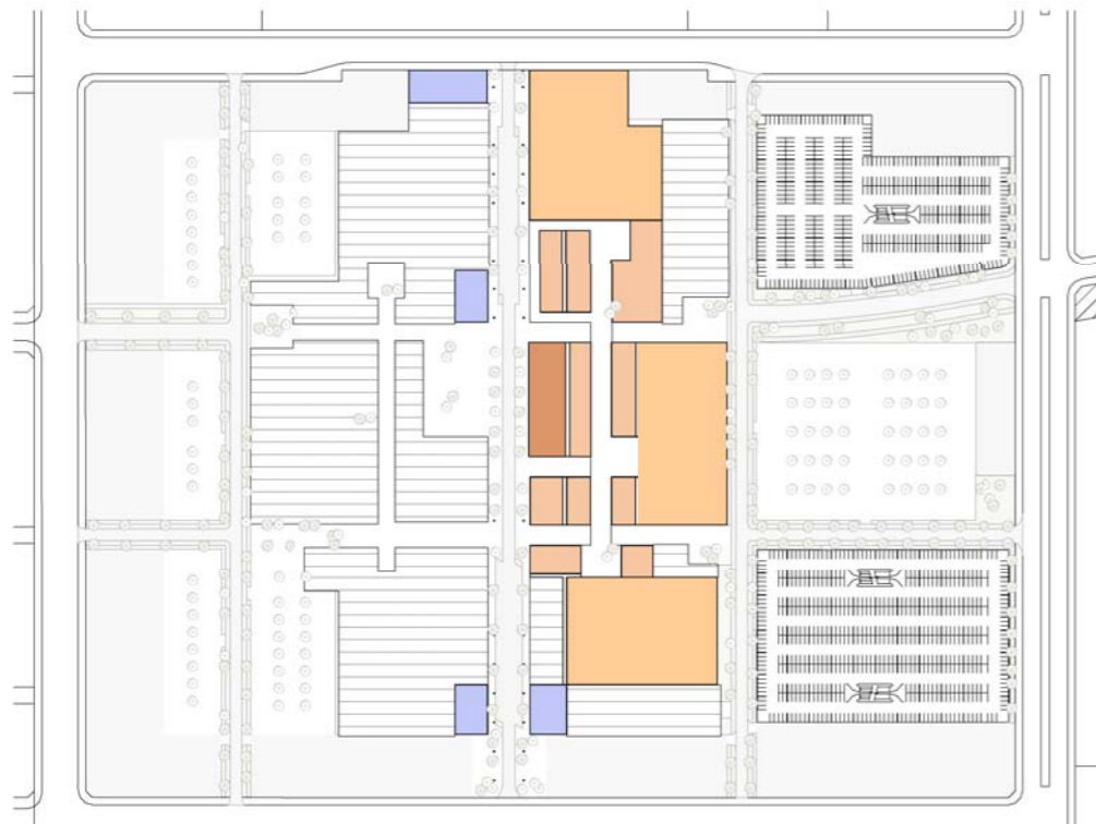
3 LEVEL 1 - GFA 1 : 2500
