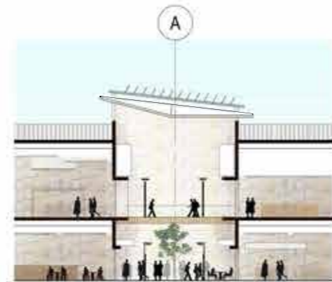
5 SECTION 5 1:250
