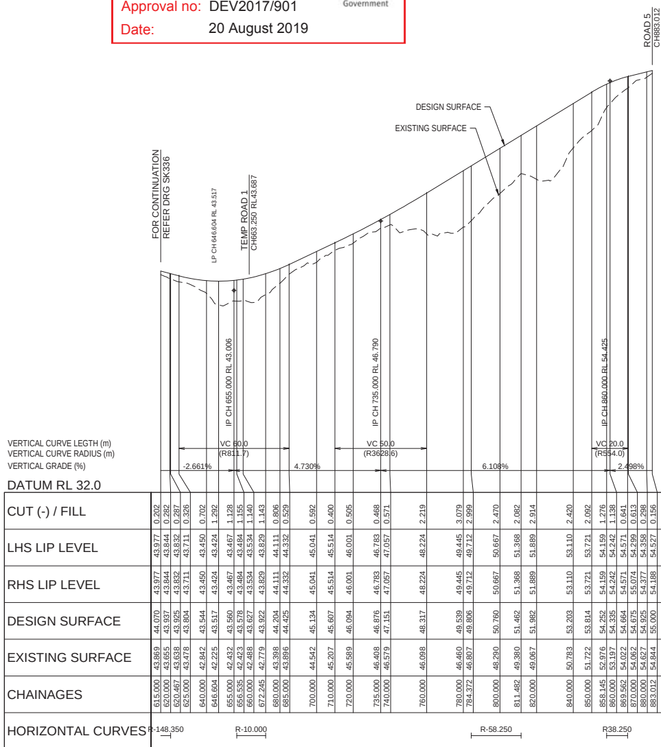
LONGITUDINAL SECTION - ROAD 5
