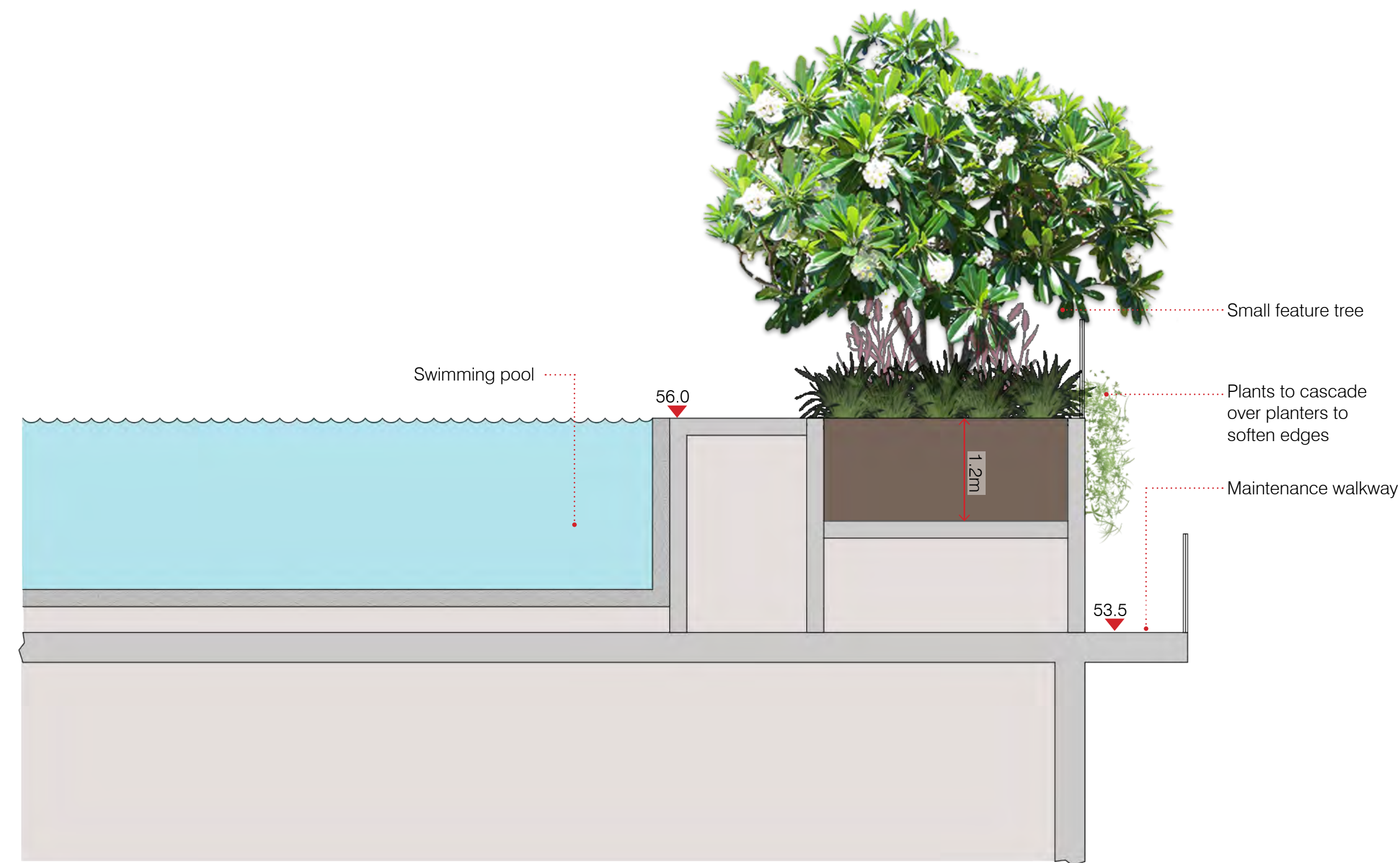
SECTION F-F 1:50 @ A1; 1:100 @ A3
