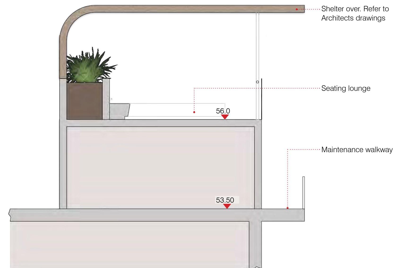
SECTION H-H 1:50 @ A1; 1:100 @ A3
