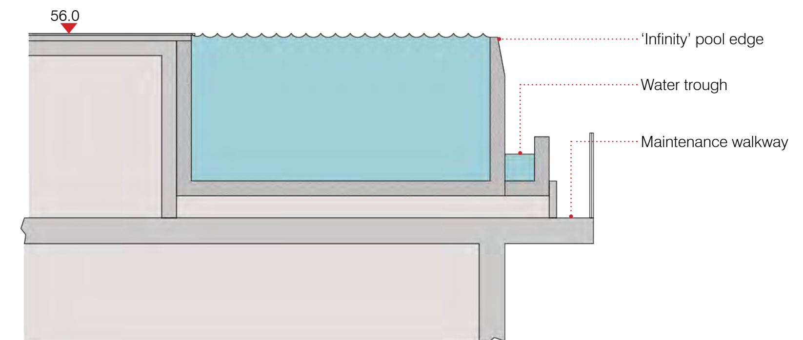
SECTION I-I 1:50 @ A1; 1:100 @ A3
