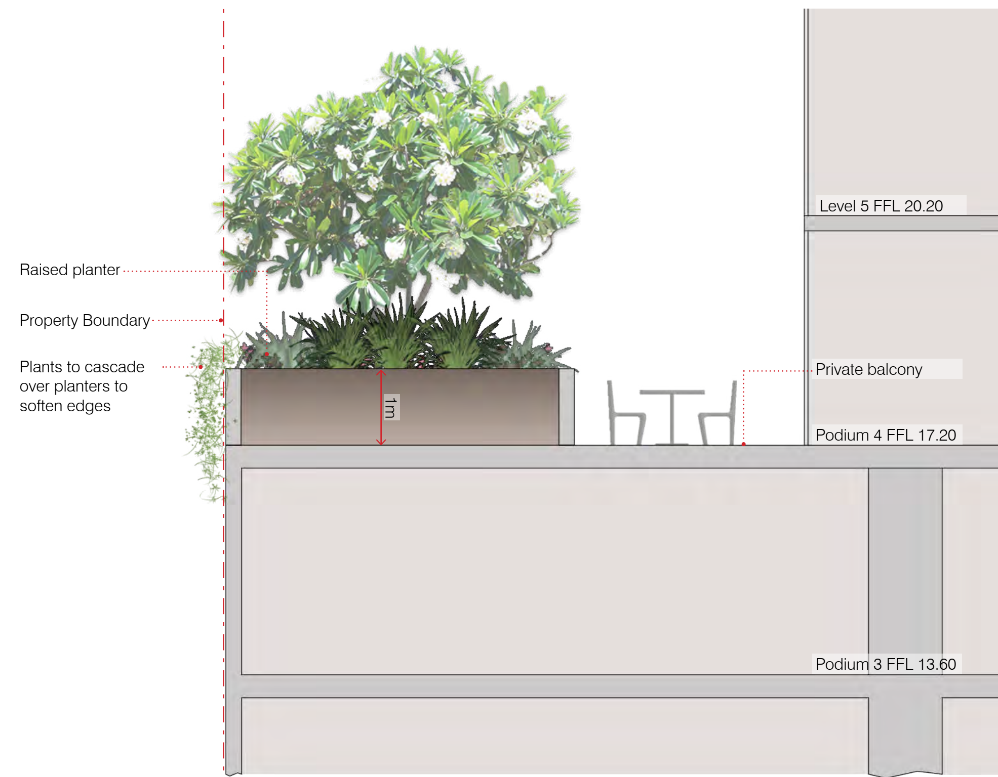
SECTION E-E 1:50 @ A1; 1:100 @ A3
