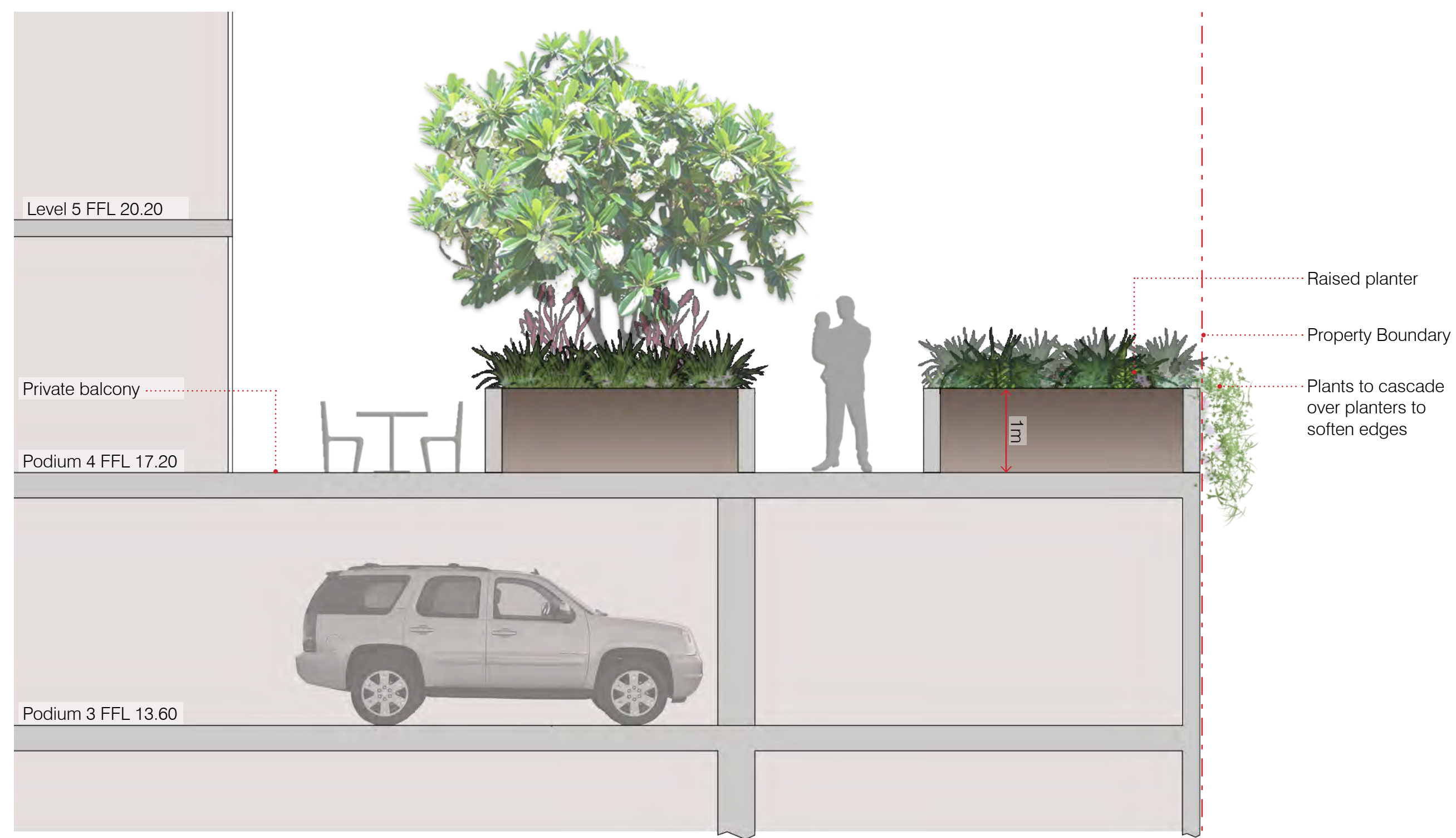
SECTION D-D 1:50 @ A1; 1:100 @ A3
