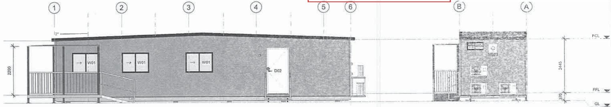
A ELEVATION A01 1:50
